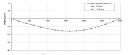
Vlakheid berekend op basis van de waterpasmetingen grafiek 5
