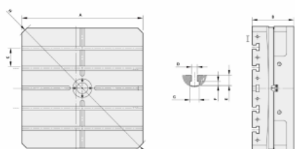
GCT 外觀尺寸對照表 | GCT DIMENSION CHART | GCT 外觀尺寸表
