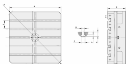
GCT 外觀尺寸對照表 | GCT DIMENSION CHART | GCT 外觀尺寸表
